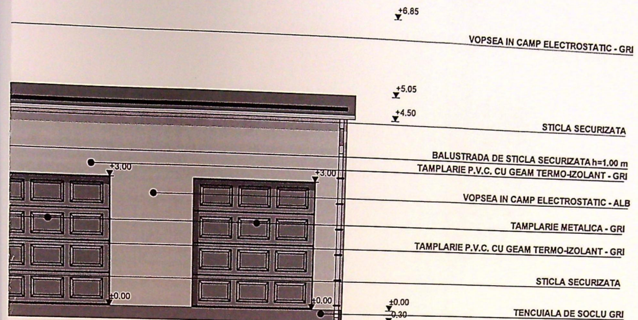
FATADA SUD
