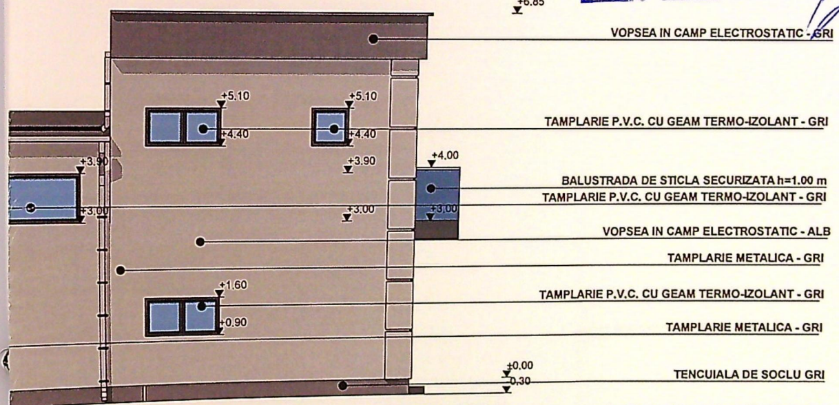
FATADA NORD
